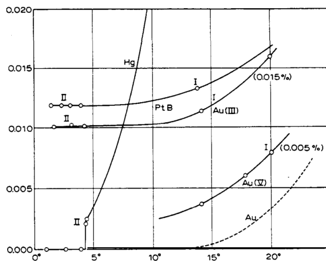
Figura 2.2 Comportamento de alguns materiais estudados por Onnes. Para a Platina, a resistência se tornou independente da temperatura. O ouro também apresentou resistência constante, e sua resistência não foi para zero mesmo na amostra pura. A linha pontilhada apresenta uma curva hipotética para o ouro puro. A curva do Mercúrio apresenta uma queda abrupta na resistência. [14]
