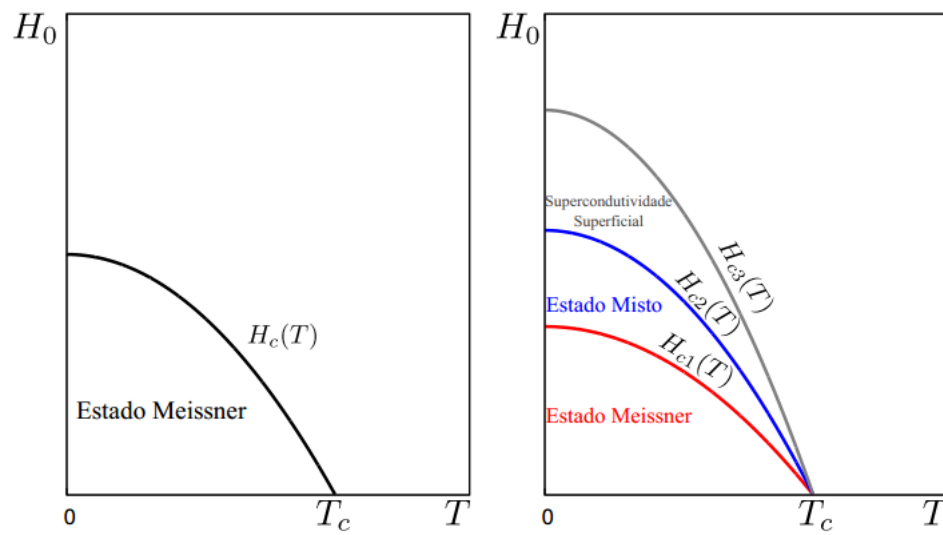
Figura 2.7 Campos críticos em função da temperatura para supercondutores do tipo-I(esquerda) e do tipo-II(direita) [22].
