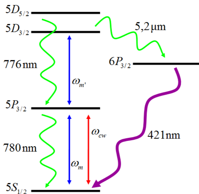
Figura 3.5: Diagrama simplificado dos níveis de energia e transições de interesse. O símbolo \omega_{cw} representa a frequência do laser de diodo, enquanto que \omega_{m'} e \omega_m representam as frequências dos modos do pente de frequências mais próximas das ressonâncias mostradas na figura. As linhas curvas representam os possíveis caminhos que o átomo pode seguir no decaimento espontâneo.
