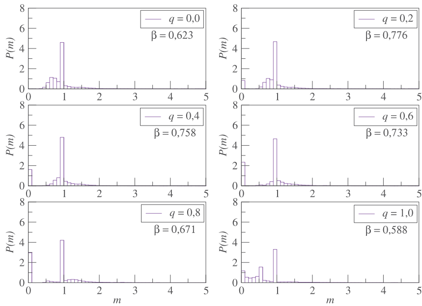
Figura 4.7: Comportamento da distribuição de renda P(m) para o modelo heterogêneo adaptativo com informação. Cada gráfico possui uma fração p = 0,8 de agentes com informação, frações q de agentes do tipo MHA2 e coeficiente de bimodalidade \beta .
