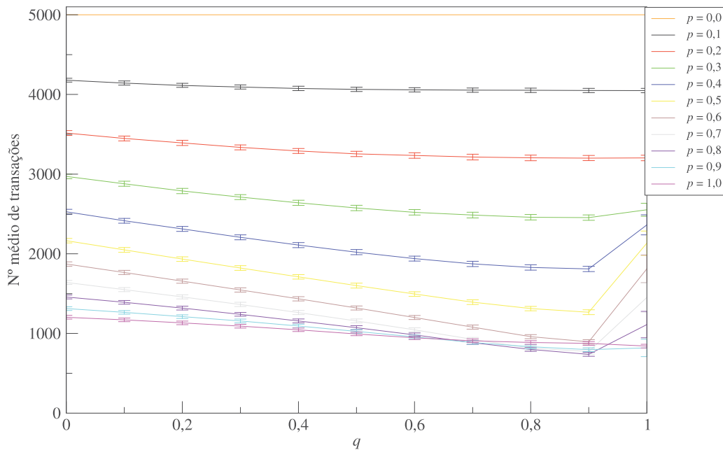
Figura 4.9: Gráfico do número médio de transações em função da fração q de agentes do tipo MHA2. As diversas cores representam a fração p de agentes com informação.
