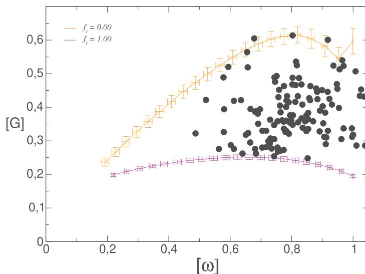
Figura 2.9: Resultados para os valores médios do coeficiente de Gini e taxa de gasto para f_r = 0 (curva laranja) e f_r = 1 (curva rosa) comparados com dados reais (círculos pretos) para 132 países, no período de 1998 à 2012. Retirada e modificada de [49].
