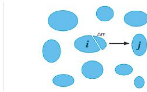
Figura 2.1: Representação esquemática da interação entre gotas de água, onde i e j representam gotas com massa m , quando as duas colidem, i perde uma quantidade \Delta m de massa que é absorvida por j . Retirada de [10].
