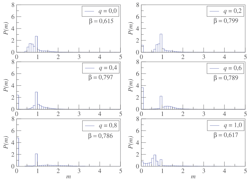
Figura 4.5: Comportamento da distribuição de renda P(m) para o modelo heterogêneo adaptativo com informação. Cada gráfico possui uma fração p = 0,4 de agentes com informação, frações q de agentes do tipo MHA2 e coeficiente de bimodalidade \beta .
