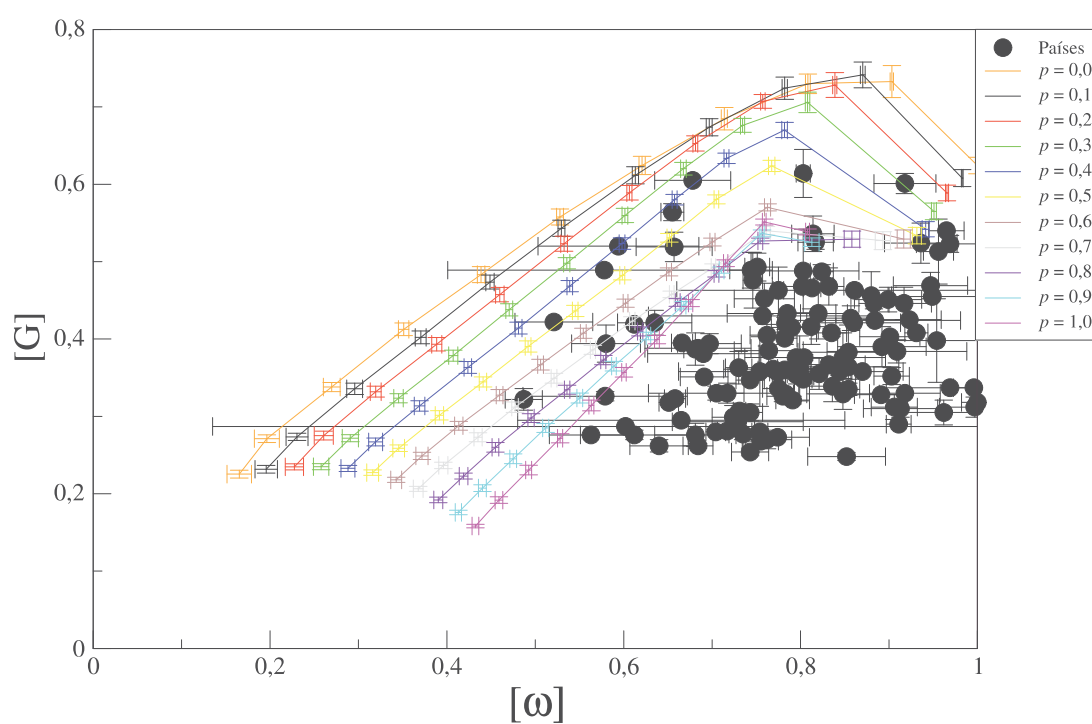
Figura 3.7: Gráfico do índice de Gini [G] da taxa de gasto [\omega] para sistemas com frações de agentes do tipo MHA2 distribuídos no intervalo 0 \leq q \leq 1 em passos dq = 0,1 , frações de agentes com informação de acordo com a legenda e dados do banco mundial referente a 123 países extraídos no período de 2000 à 2017 (círculos pretos) [13,14].
