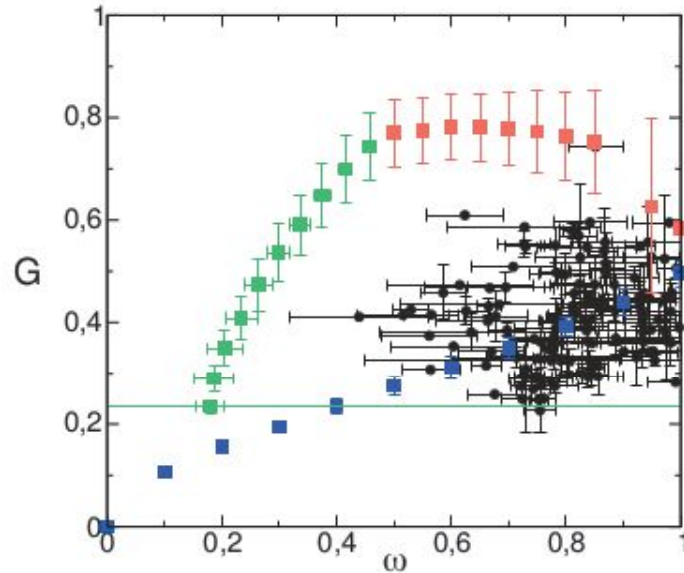
Figura 2.6: Resultados para o coeficiente de Gini e taxa de gasto do MHA1 (quadrados verdes), MHA2 (quadrados vermelhos) e modelo homogêneo (quadrados azuis) em comparação com as médias para o coeficiente de Gini e taxa de gasto de 123 países, no período de 1990 à 2009 (círculo pretos). Retirada de [10].
